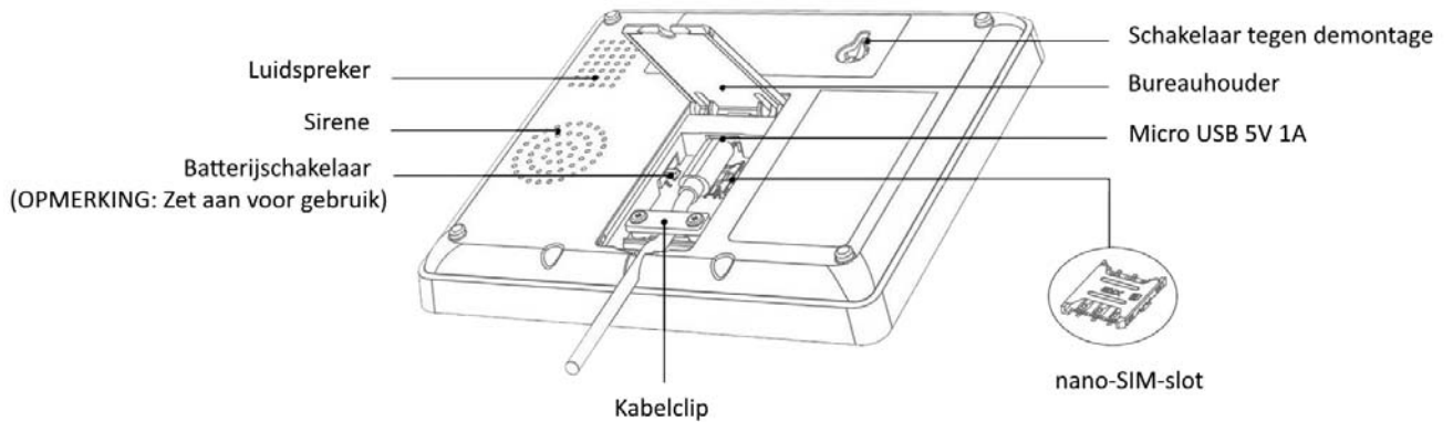
Achteraanzicht
